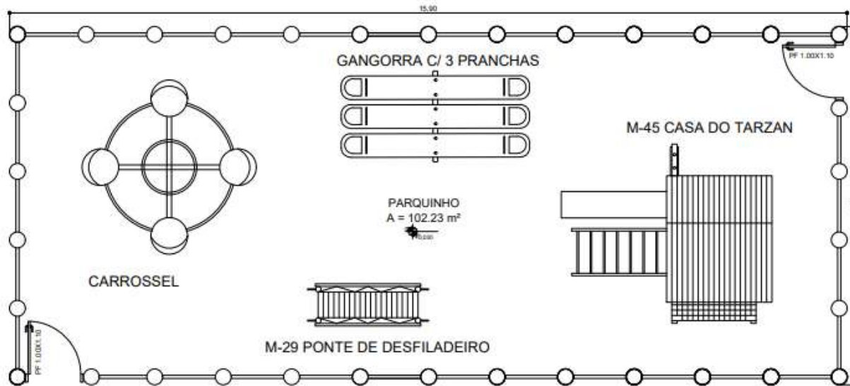
PLANTA BAIXA DO PARQUINHO O POVOADO DE CAPIM DE RAIZ
