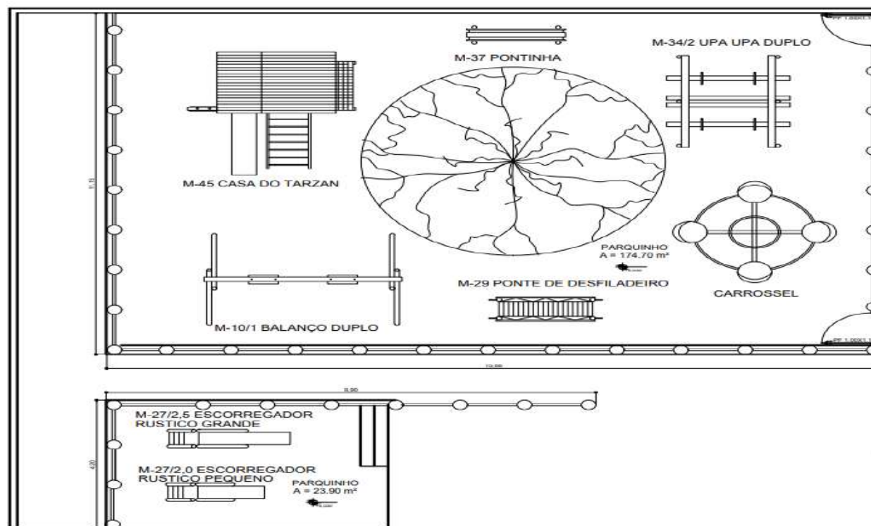
PLANTA BAIXA DO PARQUINHO ESCOLA HORÁCIO DE MATOS ESCALA: 1/100
