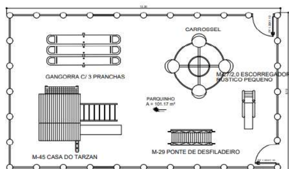
PLANTA BAIXA PARK ESCOLA AGENOR LEITE ESCALA: 1/100
