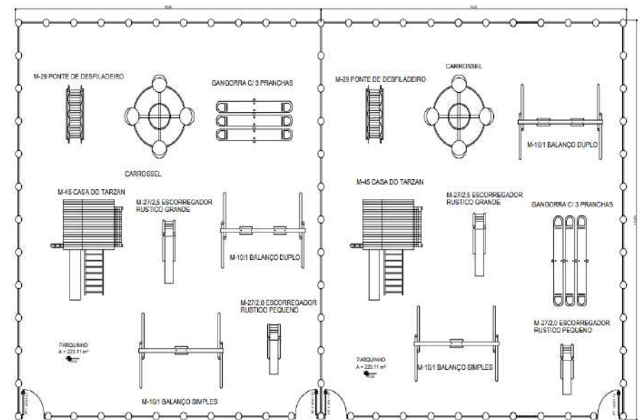
PLANTA BAIXA DO PARQUINHO DA CRECHE ESCALA: 1/100
